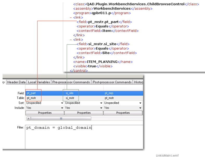
Fig. 4.9 XML Fields
