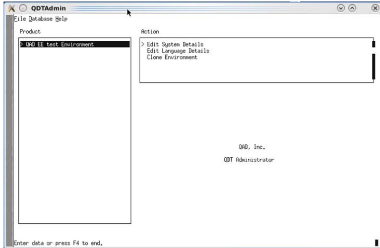
Fig. 9 QDTAdmin Screen
