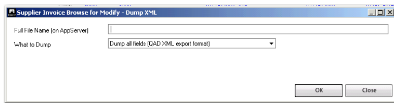
Fig. 4.20 Dump XML
