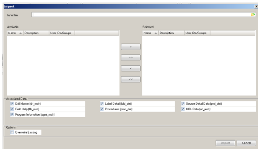
Fig. 4.31 Browse Import
