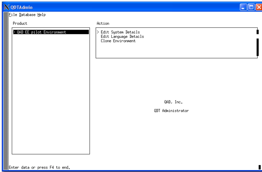
Fig. 4.4 QDT Admin
