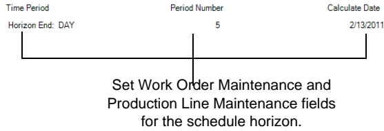
Fig. 2.9 Preferences
