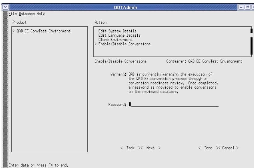
Fig. 3.3 Enable Conversions
