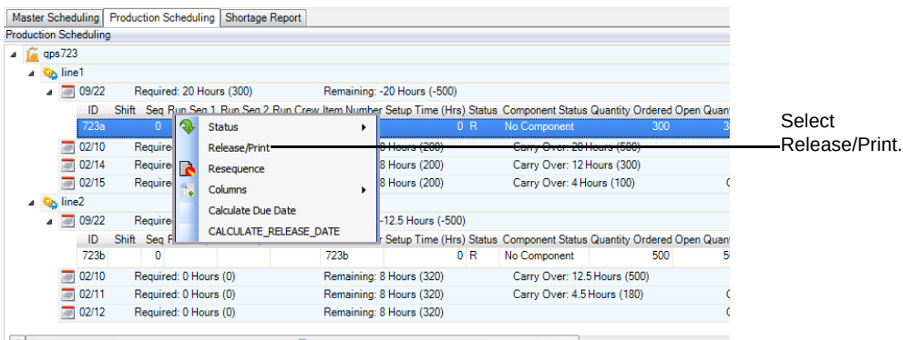
Fig. 3.13Y Print Function
