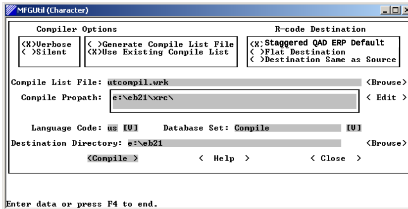
Fig. 6.8 MFG/UTIL Compiler
