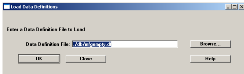
Fig. 3.8 Loading mfgempty.df
