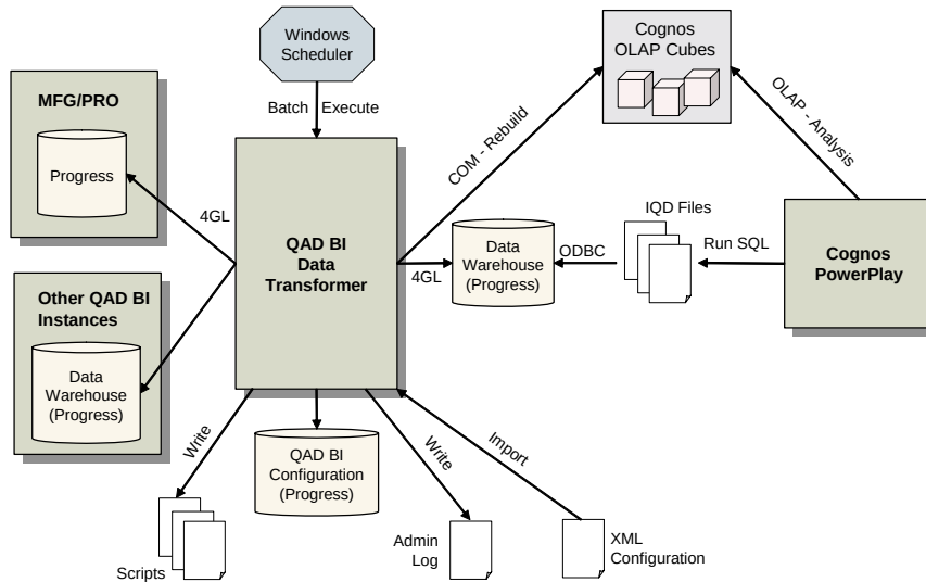
Fig. 3.1 QAD BI Overview
