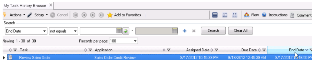
Fig. 2.48 End Date
