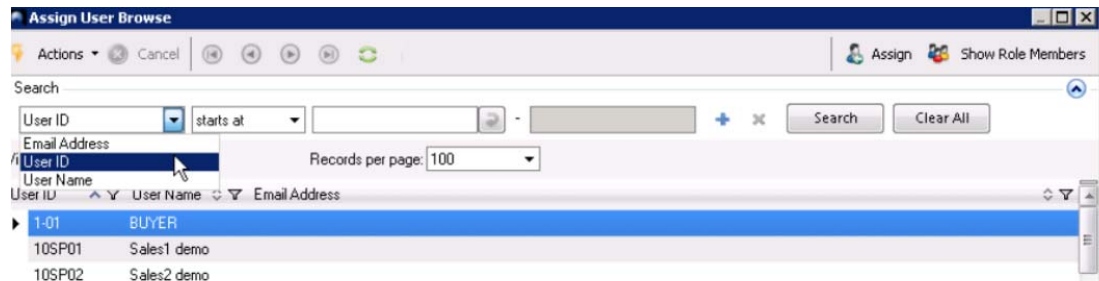
Fig. 2.48
