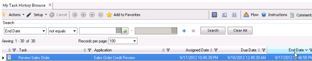
Fig. 2.49 End Date
