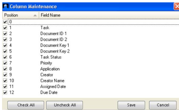
Fig. 2.65 Display Columns
