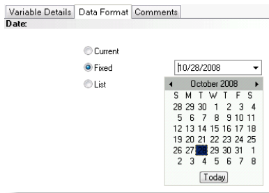
Fig. 5.11 Date Format
