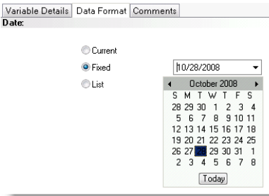
Fig. 5.11 Date Format
