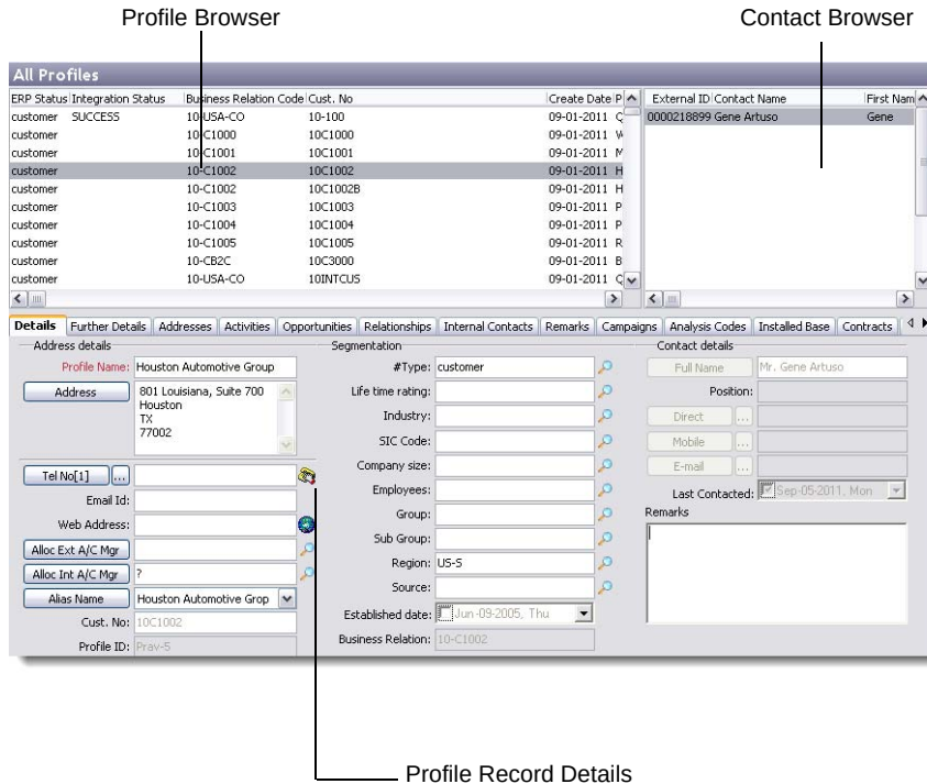
Fig. 7.3 All Profiles
