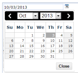
Fig. 1.4 Calendar
