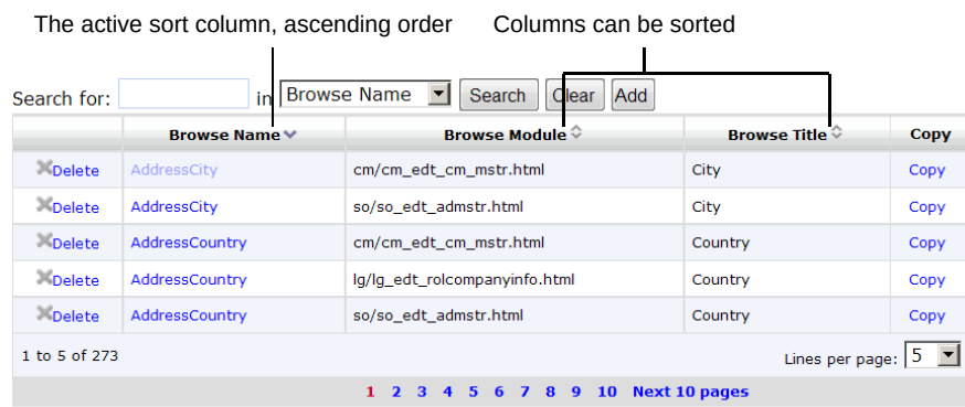
Fig. 1.8 Sorting Columns
