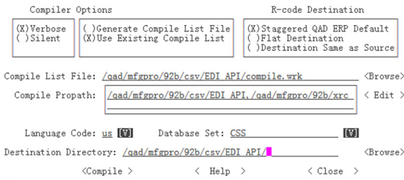
Fig. 2.25 Compile EDI_API
