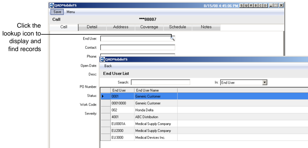
Fig. 2.3 Using Lookups
