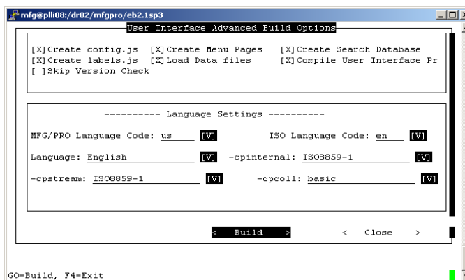
Fig. 9.2 Default Values for English
