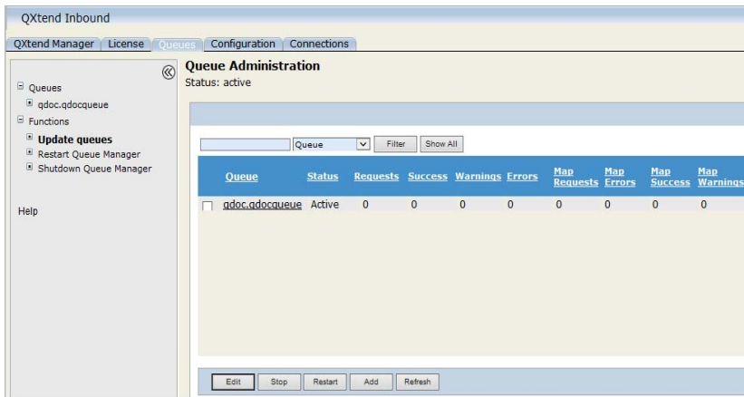
Fig. 15.10 Update Queue
