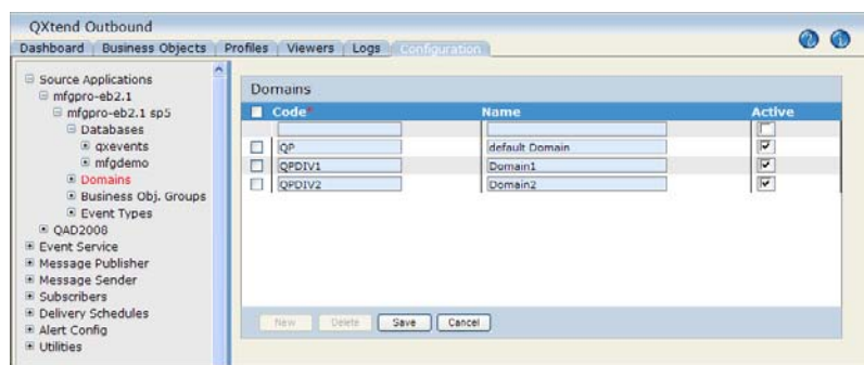
Fig. 2.6 Domains
