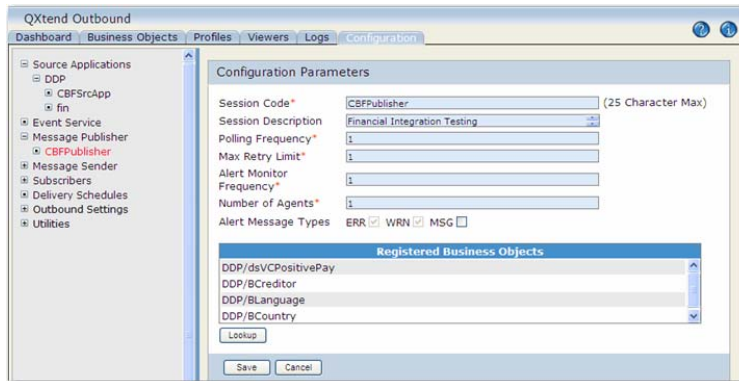
Fig. 11.11 Message Publisher
