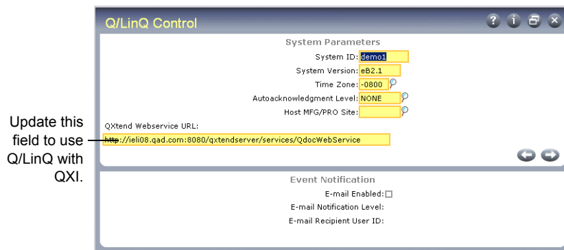
Fig. 21.1 Q/LinQ Control (36.8.24), QXtend Webservice URL
