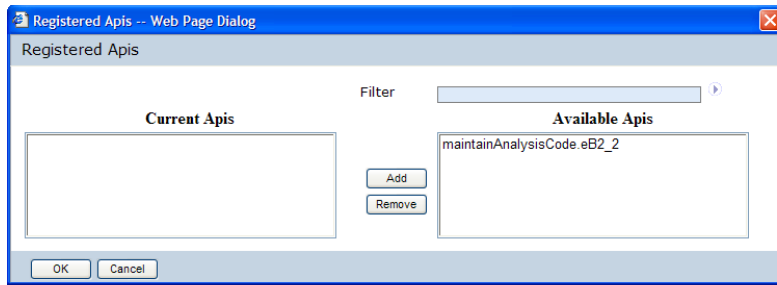
Fig. 16.32 Register APIs
