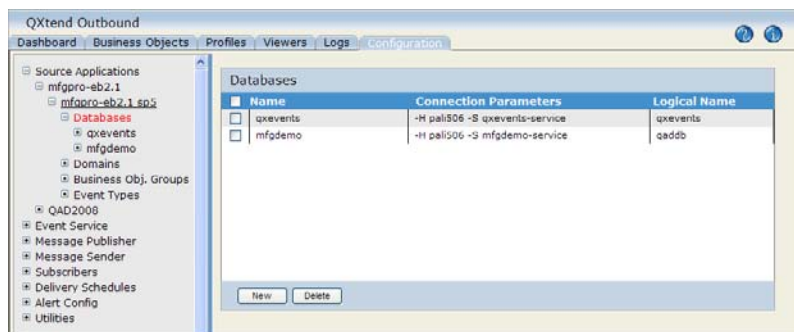
Fig. 2.4 Databases
