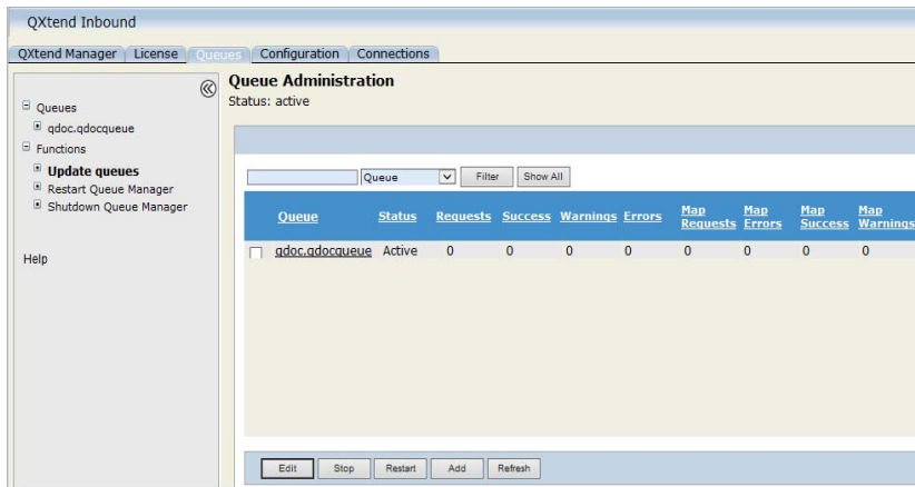
Fig. 15.10 Update Queue
