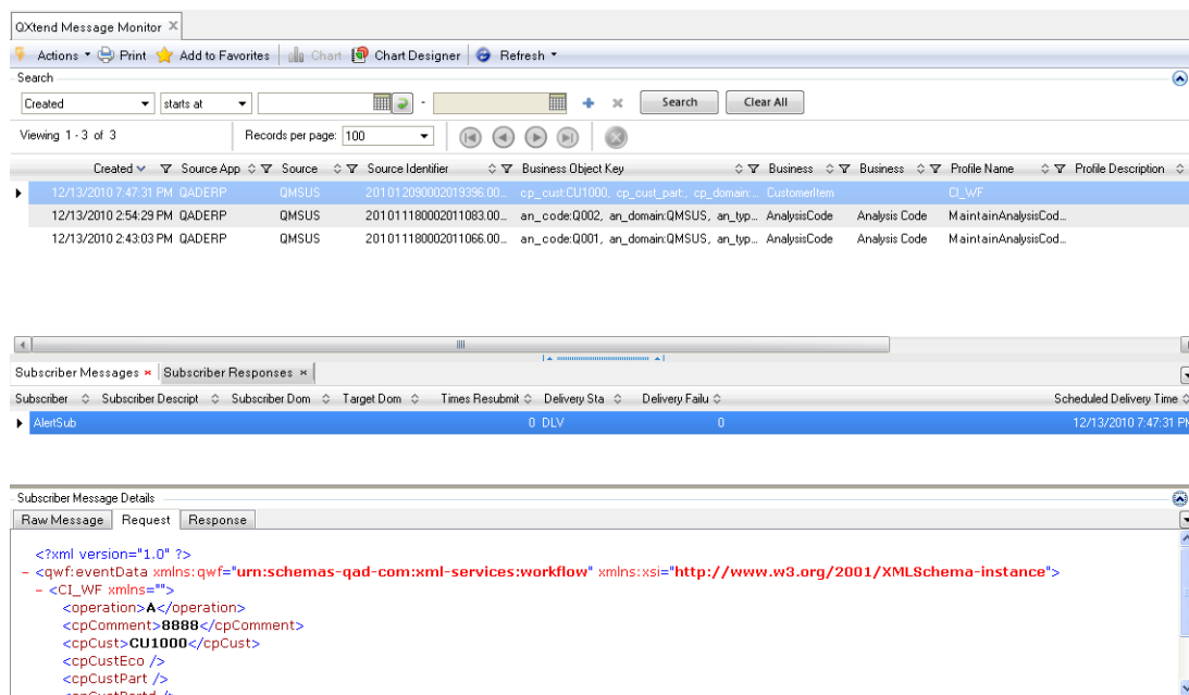
Fig. 9.1 QXtend Message Monitor
